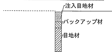
【中央部】縦目地施工参考図 N.S
