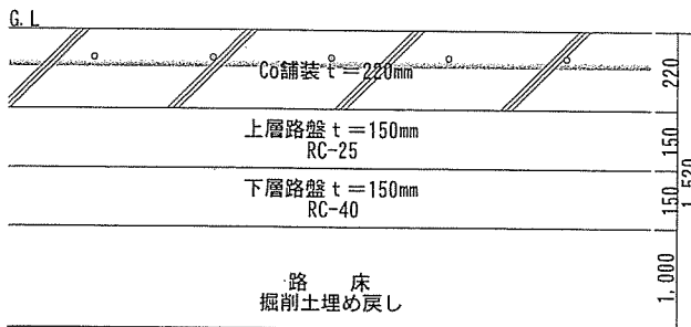
【新設】掘削断面図 N.S
