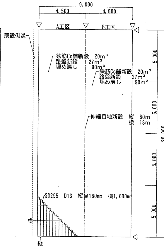
【撤去】施工詳細図 S=1/150
