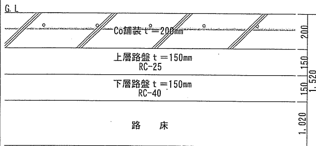
【撤去】掘削断面図 N.S
