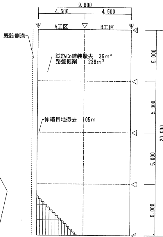
【撤去】施工詳細図 S=1/150
