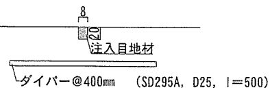
【中央部】縦目地施工参考図 N.S
