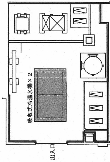
機械室配置図
