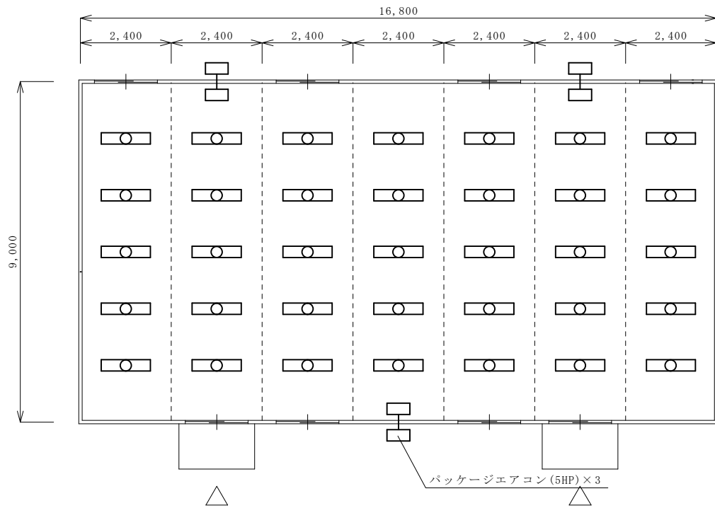
平面標準図 (A~C棟) S=1:100
