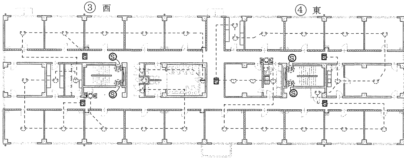
2階 平面図 s=1:x
