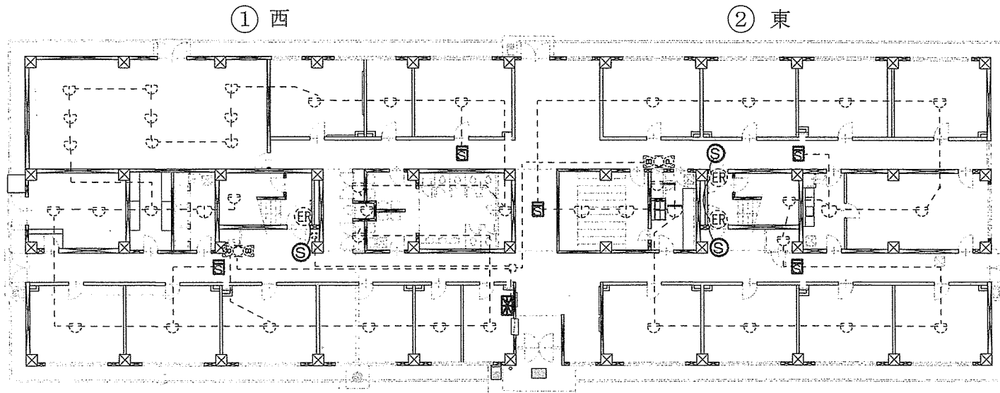
1階 平面図 s=1:x
