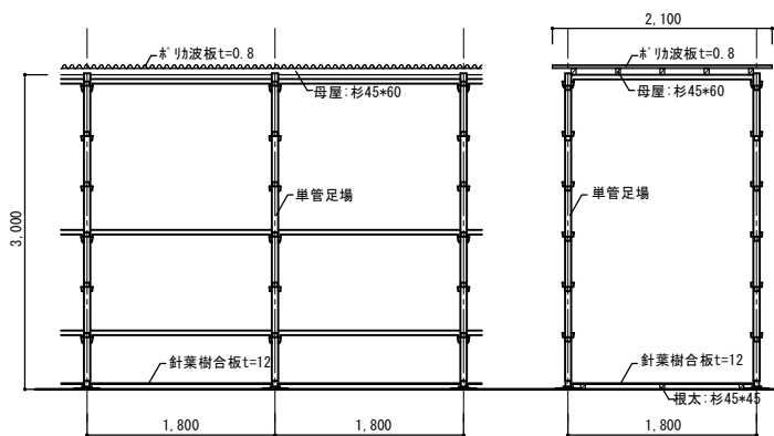
(参考図) 仮設渡り廊下詳細図 ※外部階段4階仮設屋根も同様(床合板等はなし)
